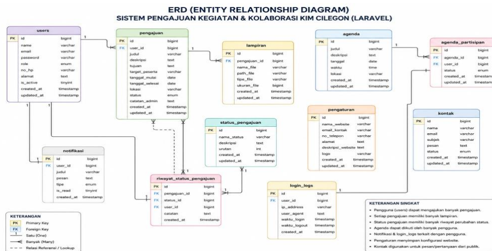
Gambar 2. Gambar ERD
