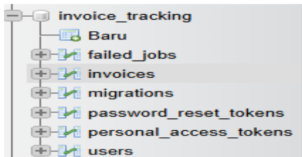
Gambar 12. ERD Sistem
