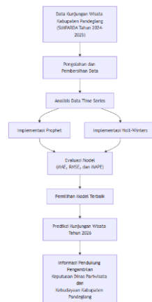
Gambar 1. Tahapan Penelitian
